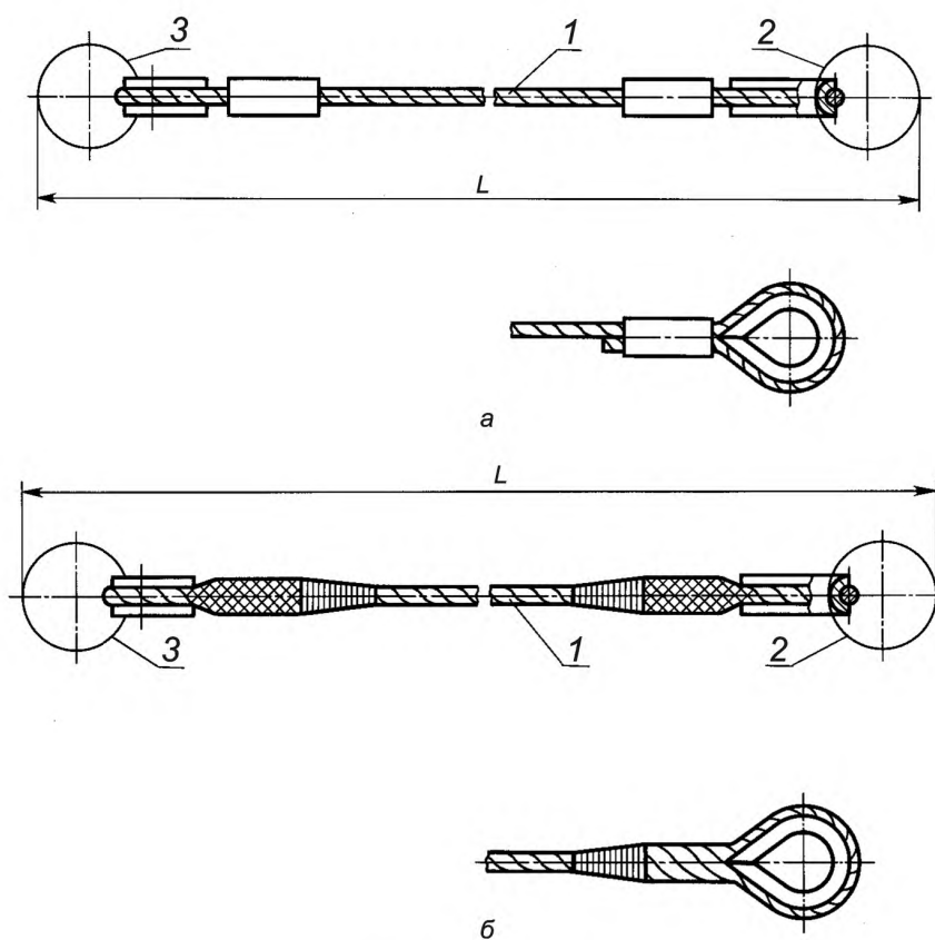
1 — канатная ветвь; 2 — звено; 3 — захват
