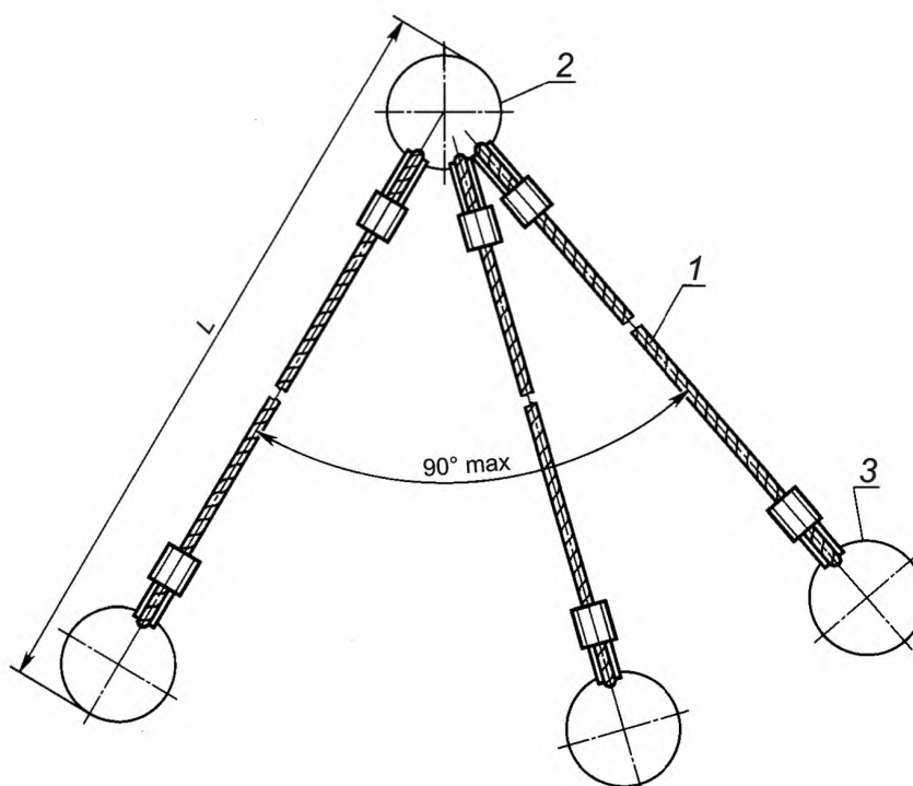
Рисунок 3 — Трехветвевый канатный строп
