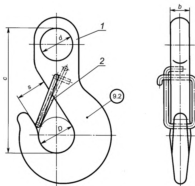
Рисунок Б.34 — Зацепной захват в виде крюка исполнения К2
