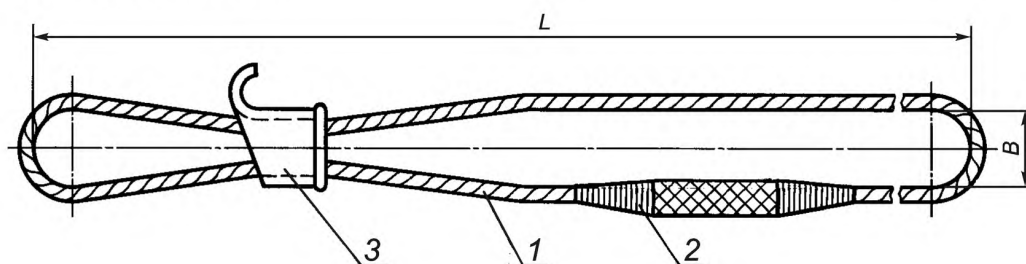
Рисунок 9 — Кольцевой канатный строп исполнения 2
